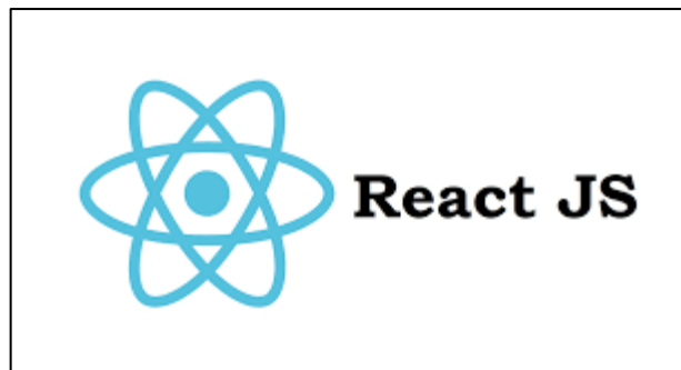
Hình 2. 1 Logo ReactJS
